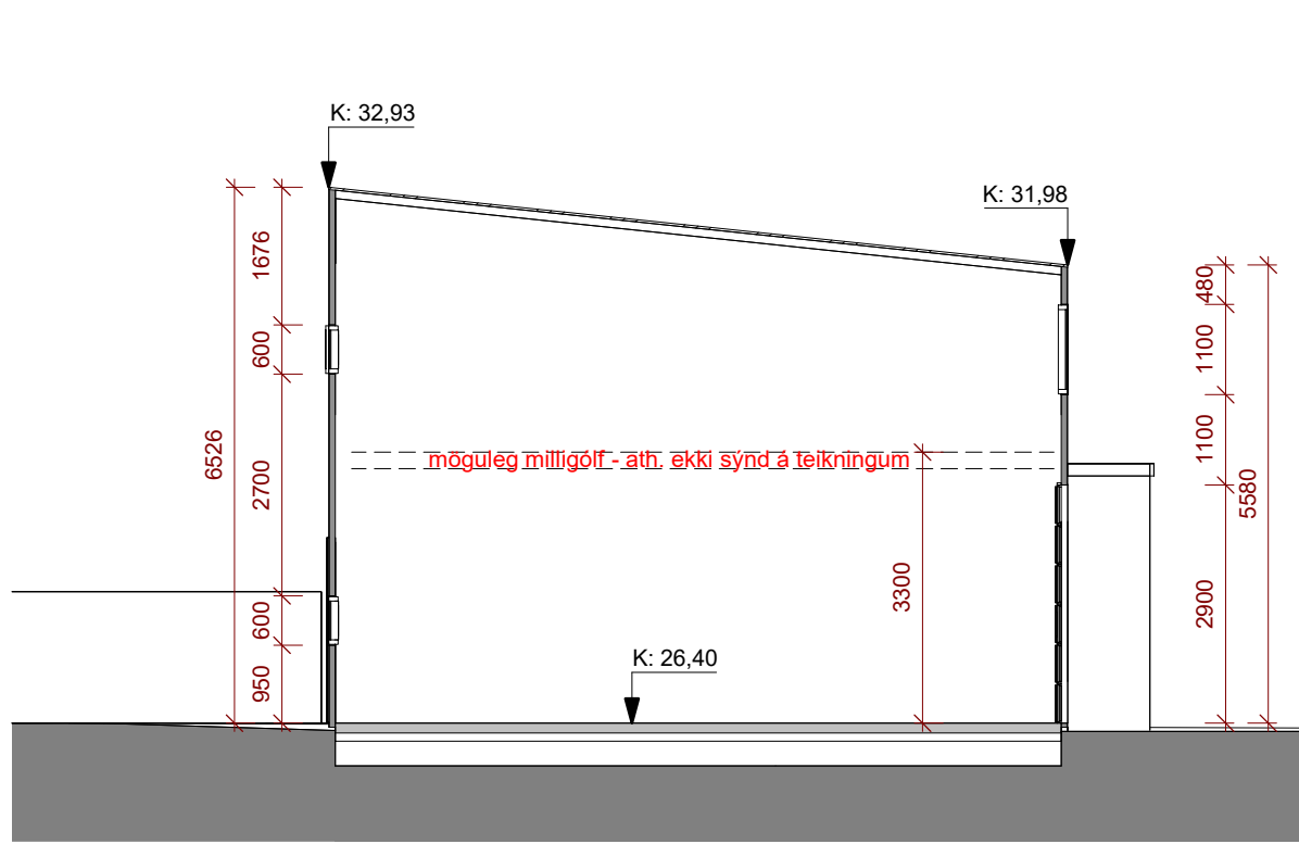
mhl 03 snið A 1 : 100
