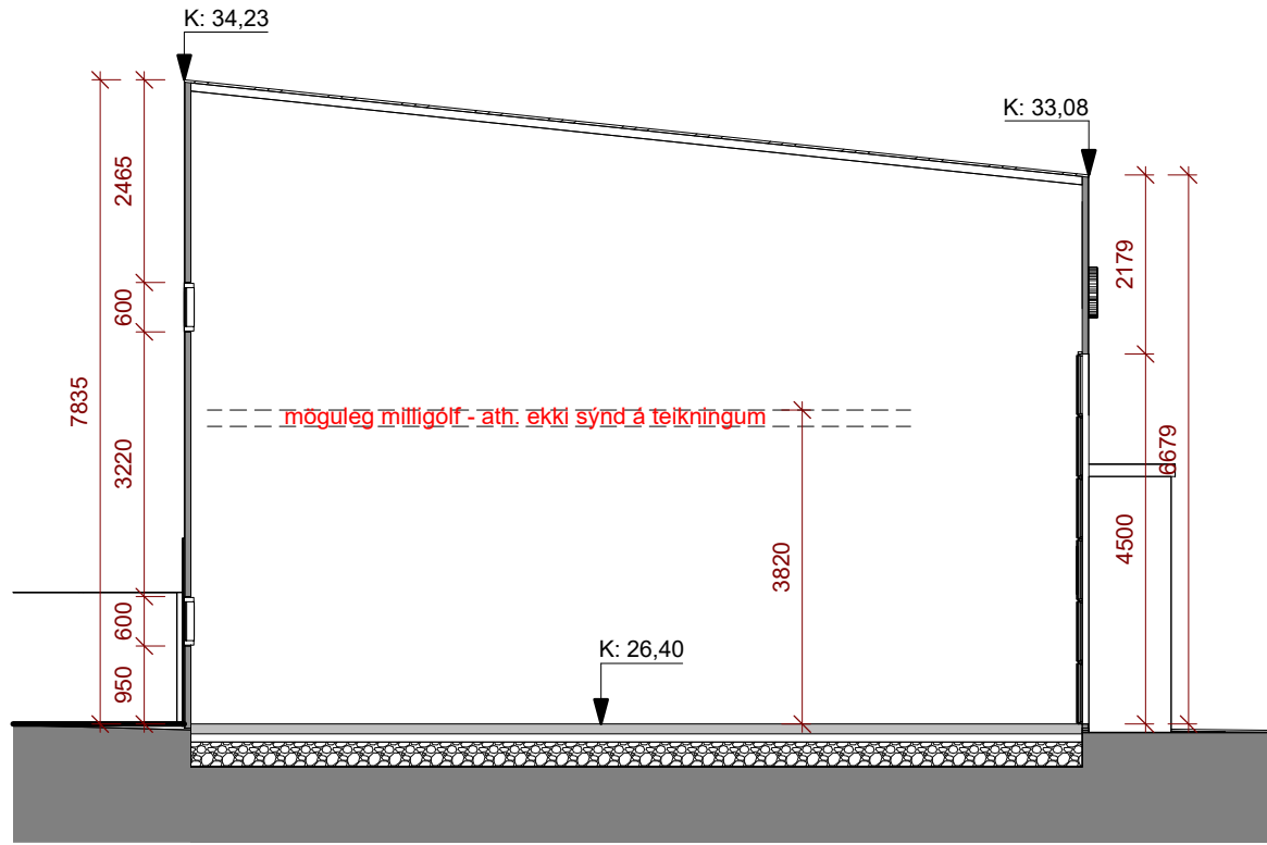
mhl 03 snið B 1 : 100
