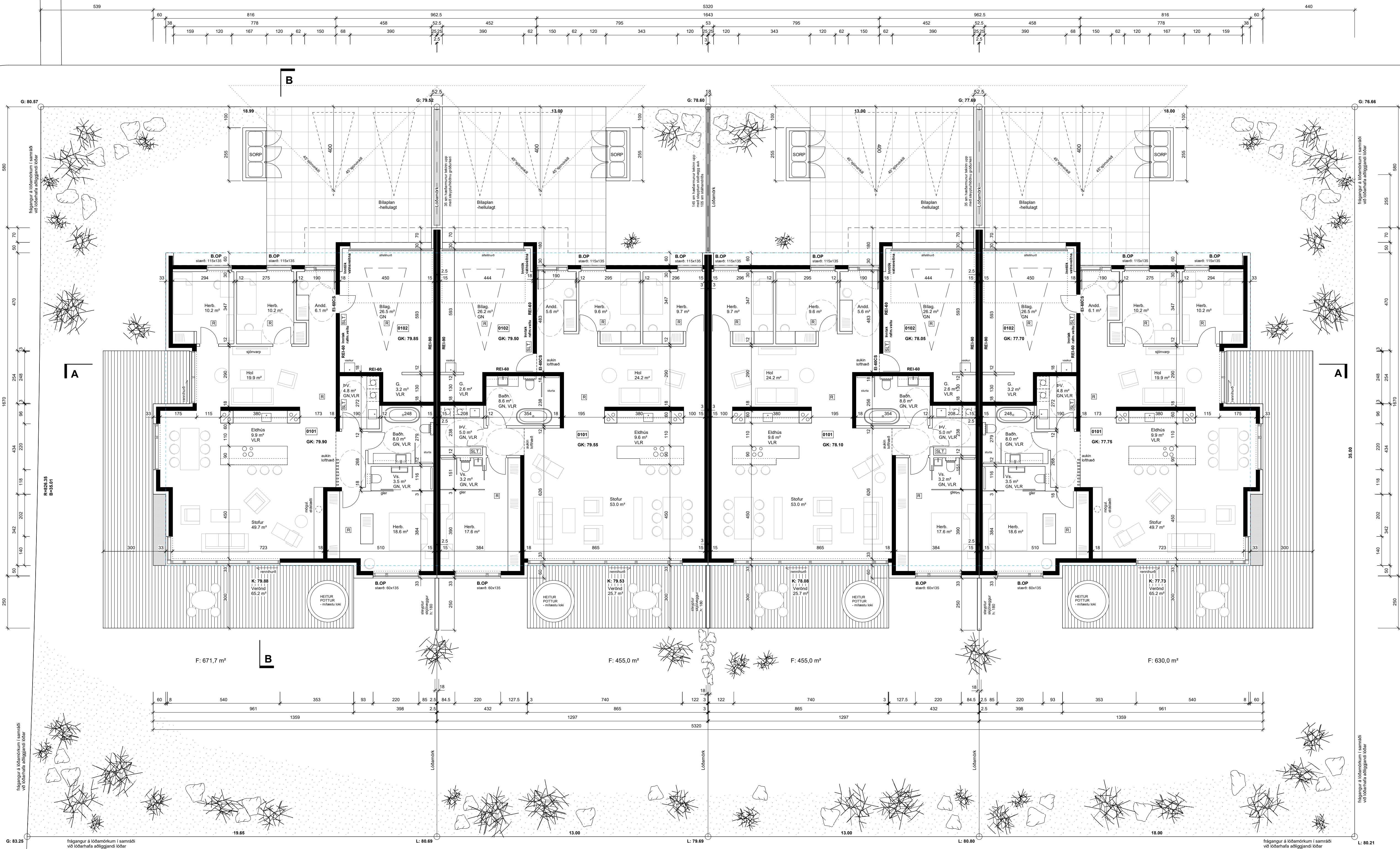
GRUNNMYND 1. HÆÐAR
